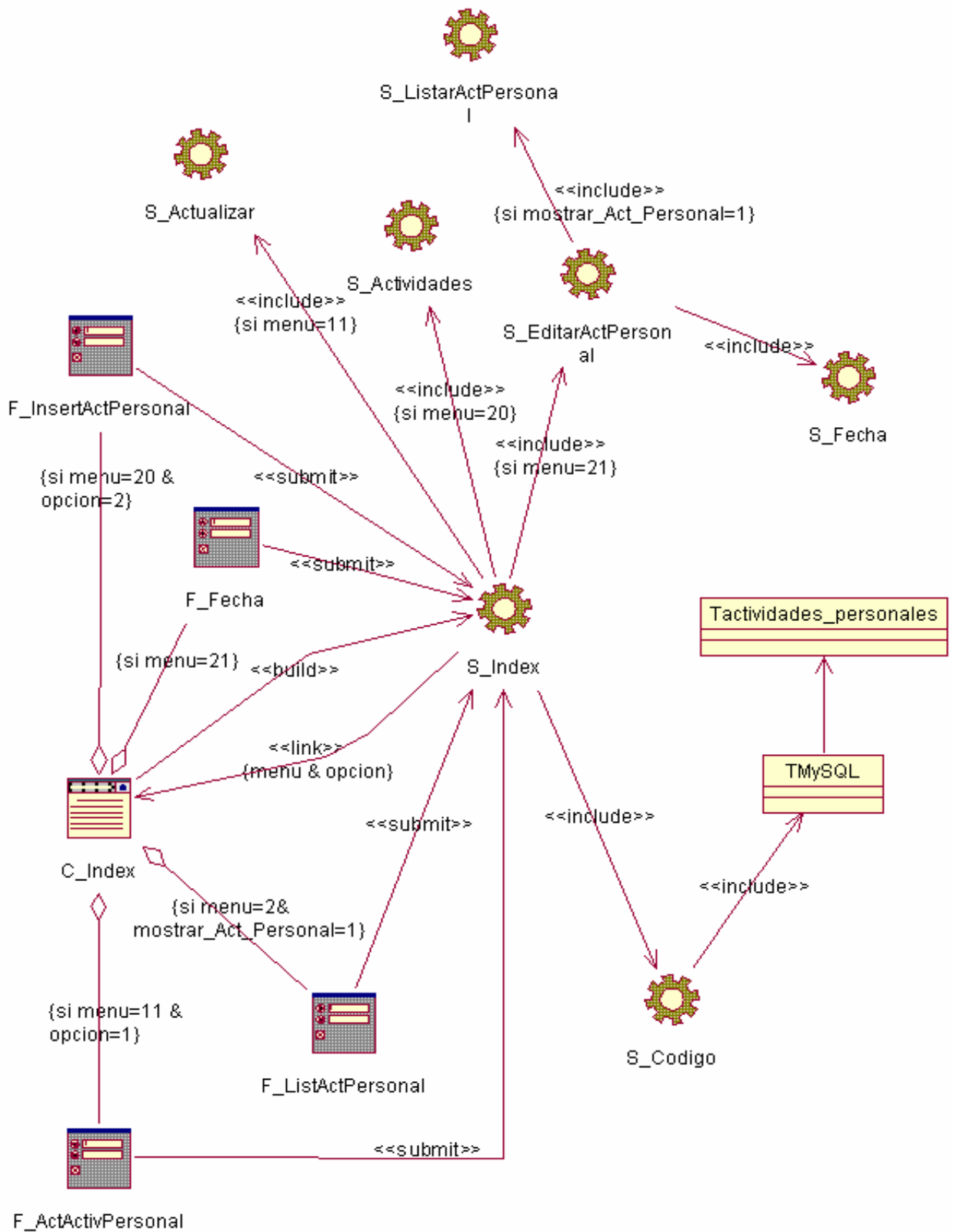
Figura 17. Modificar plan personal.
