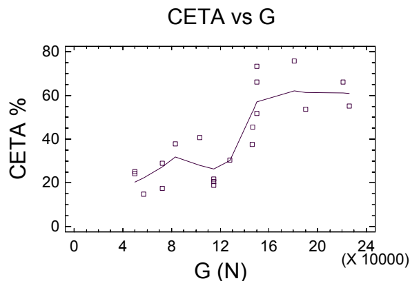
Figura 4.10. CETA vs. Peso total.
