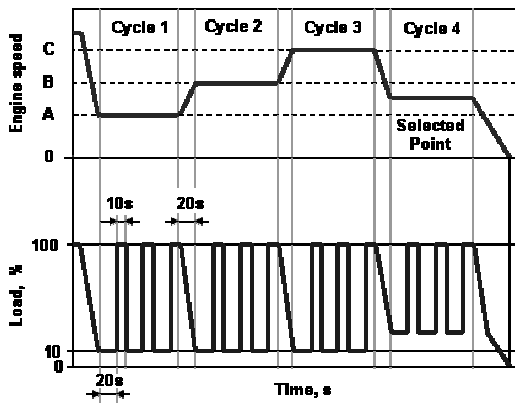
Figura 35. ELR Test
