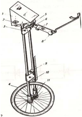
Figura 48. La quinta rueda tipo Peisler [19] .
