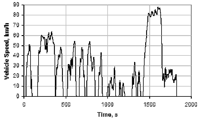
Figura 42. Ciclo JE05
