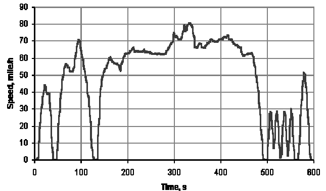
Figura 4. Ciclo SFTP US06
