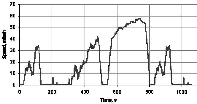
Figure 15. HD UDDS Cycle
