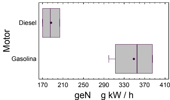
Figura 3.2. Diagrama de cajas g_{eN} vehículos pesados analizados.
