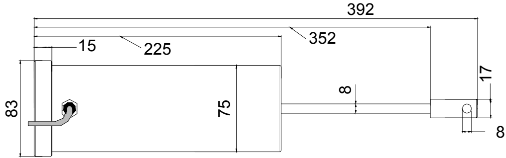
Figura 1. Sensor de desplazamientos.
