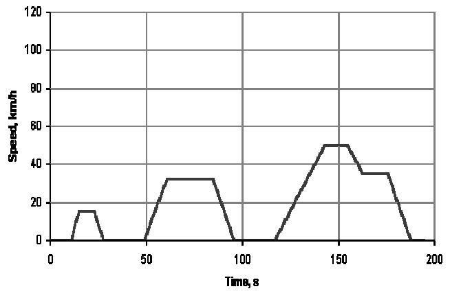
Figura 30. ECE 15 Cycle
