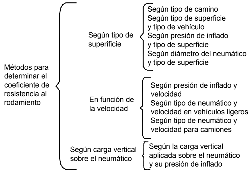
Figura 1.5 Métodos para obtener el coeficiente de resistencia al rodamiento [196] .
