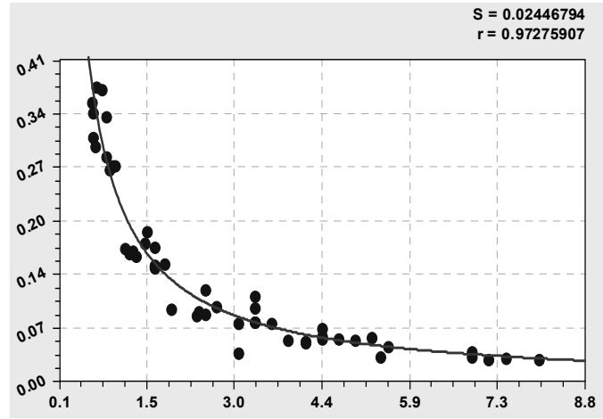
Fig. 2.3 Dependencia de \psi = f(v) : enfoque teórico (a) y determinación experimental (b).
