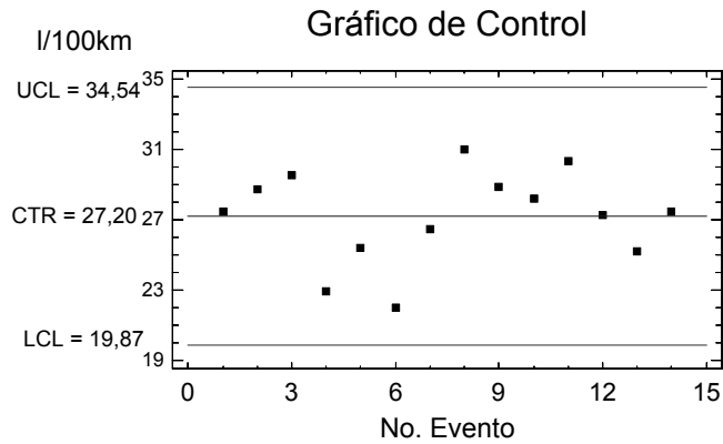
Figura 10. Gráfico de control: Consumo recorrido (actualizado en las pruebas de consumo), ómnibus MB O 371 en la ruta Cienfuegos-Habana.
