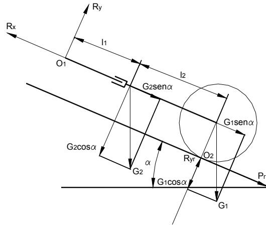
Figura 3.2. Esquema de análisis de la 5ta rueda.
