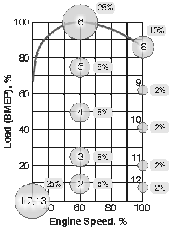
Figura 33. ECE R49 Cycle
