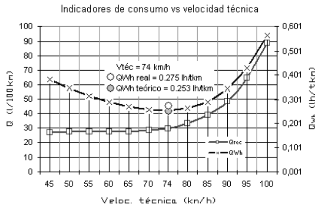
Figura 4. 9. Indicadores de consumo versus velocidad técnica.
