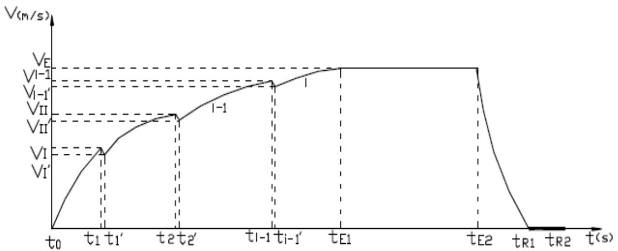
Figura 44. Ciclo Básico de movimiento [122] [140] .
