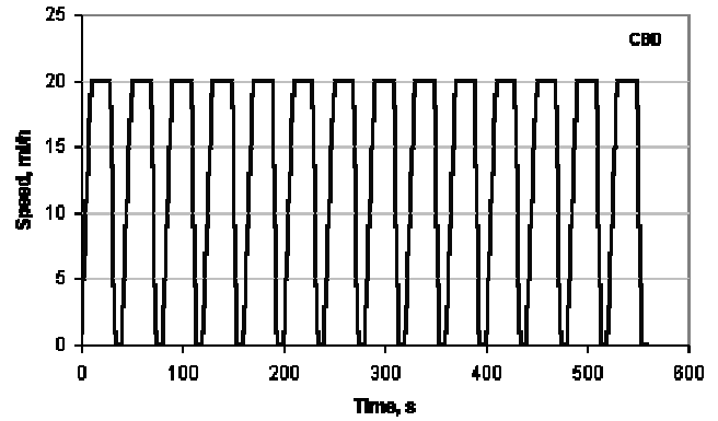
Figure 16. Ciclo de Manejo CBD
